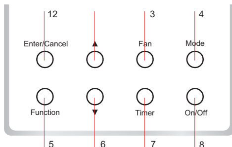
Рисунок 3 Кнопки на проводном пульте дистанционного управления
