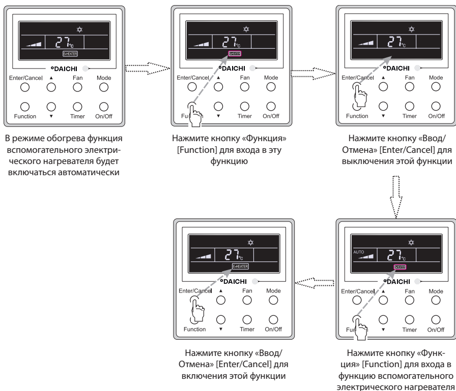
Рисунок 12 Настройка электрического нагревателя
